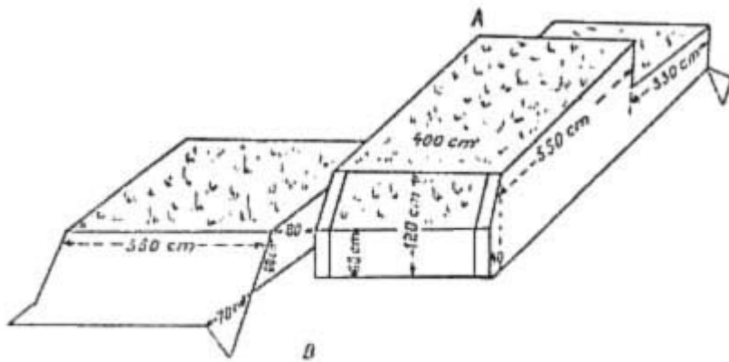
Ryc. 33. Nasyp widziany z przeciwnej strony.
