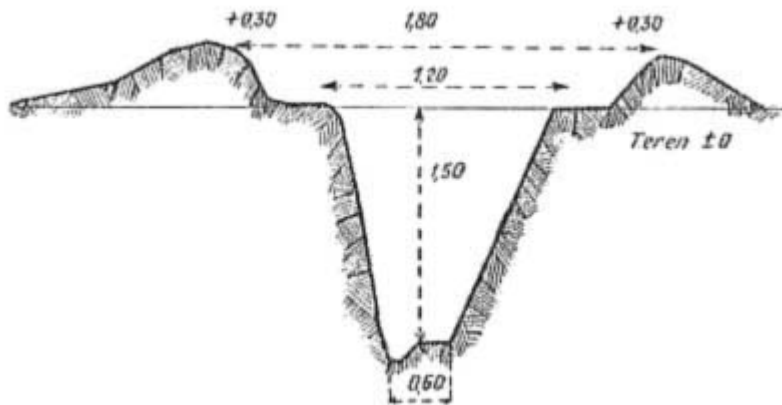
Ryc. 38. Rów łącznikowy.
