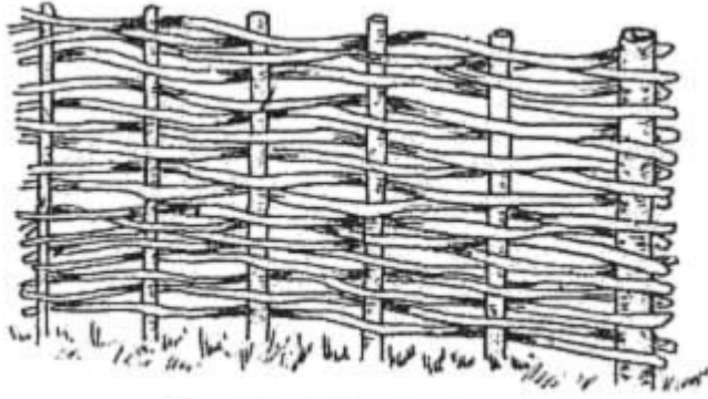
Ryc. 27. Plot pleciony.
