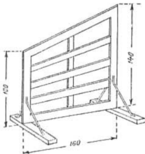
Ryc. 41. Odkos.
