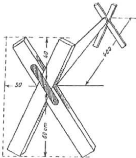
Ryc. 40. Kozioł.
