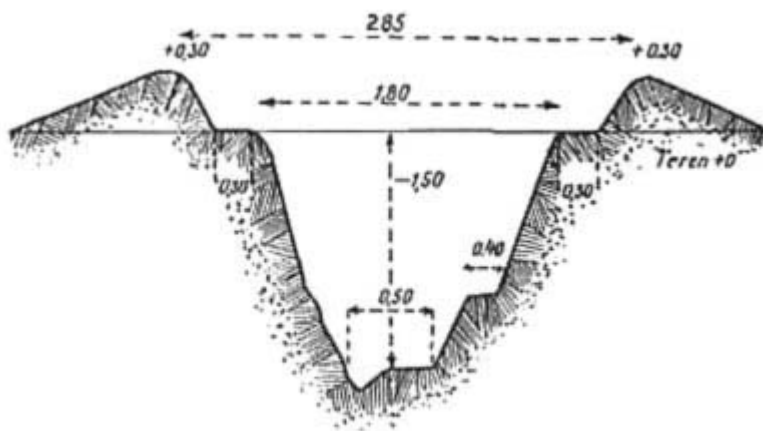
Ryc. 36. Rów strzelecki (przekrój).
