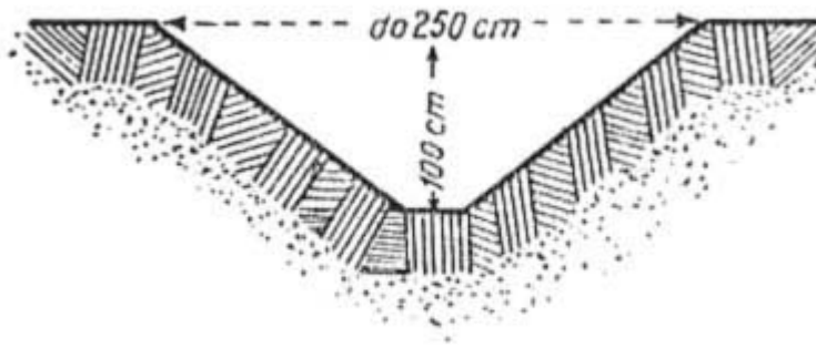
Ryc. 31. Otwarty rów.
