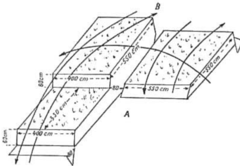
Ryc. 32. Nasyp.
