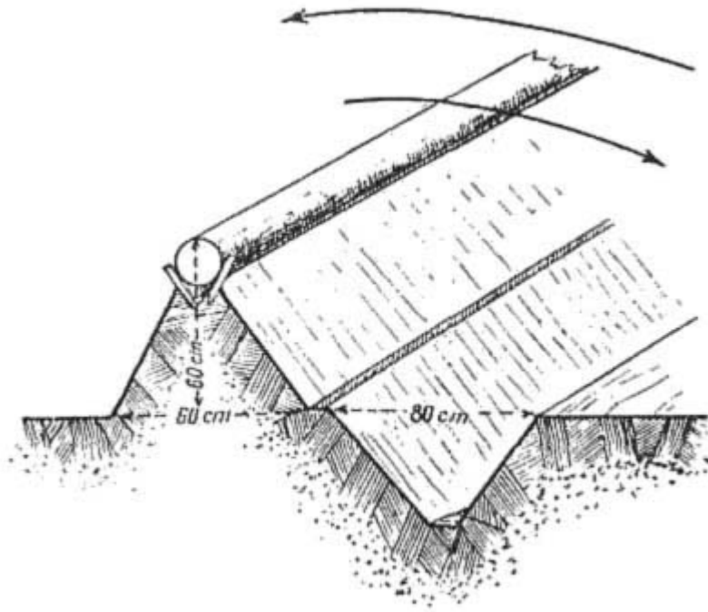
Ryc. 34. Wał ziemny z rowem.
