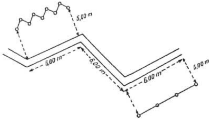
Ryc. 37. Rów strzelecki widziany z góry.
